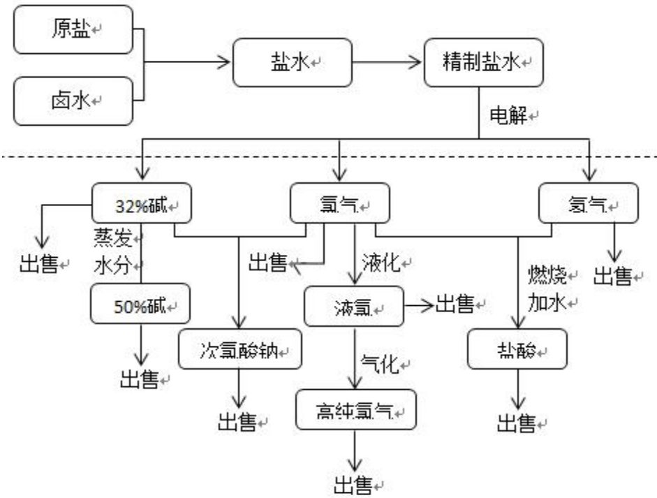
图5-3 离子膜烧碱项目生产工艺流程图
