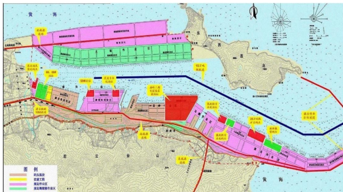
图 5-6：连云港区泊位示意图
