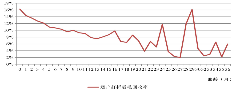
信用卡透支资产池的账龄与回收率的关系图
