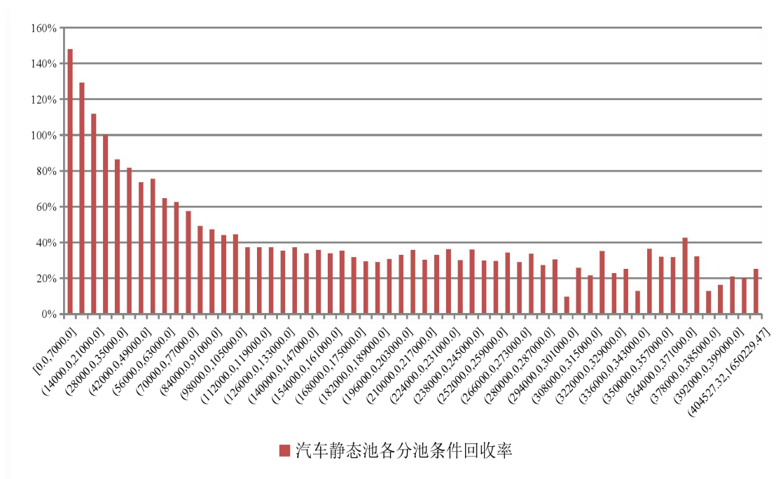
图一：汽车分期静态池分组 36 个月回收率
