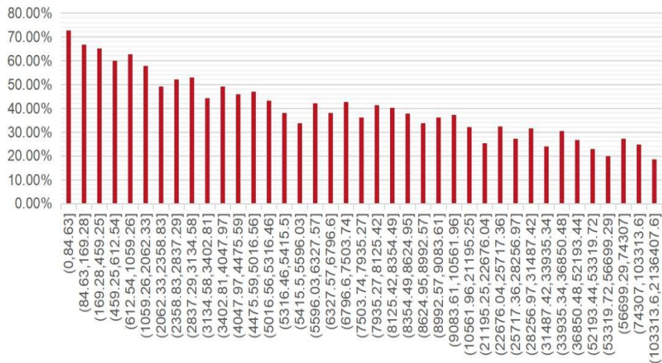
信用卡普通透支不良贷款静态样本池的 36 期回收比率表现（单位：元）
