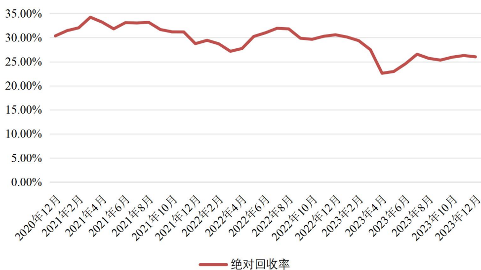
图 4 信用卡透支分期静态池各年月 24 期回收率
