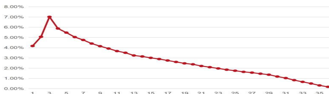
入池资产 36 期回收时间分布图（单位：月）
