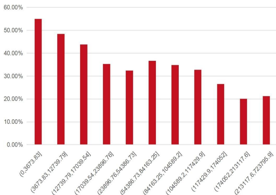
信用卡专项分期不良贷款静态样本池的 36 期回收比率表现（单位：元）
