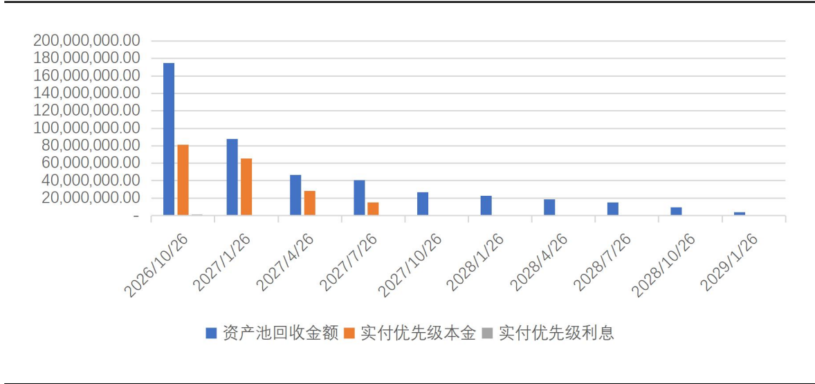
图 基准情形下优先档现金流匹配情况（单位：万元）
