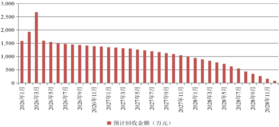
资产池预计整体回收分布图（万元）
