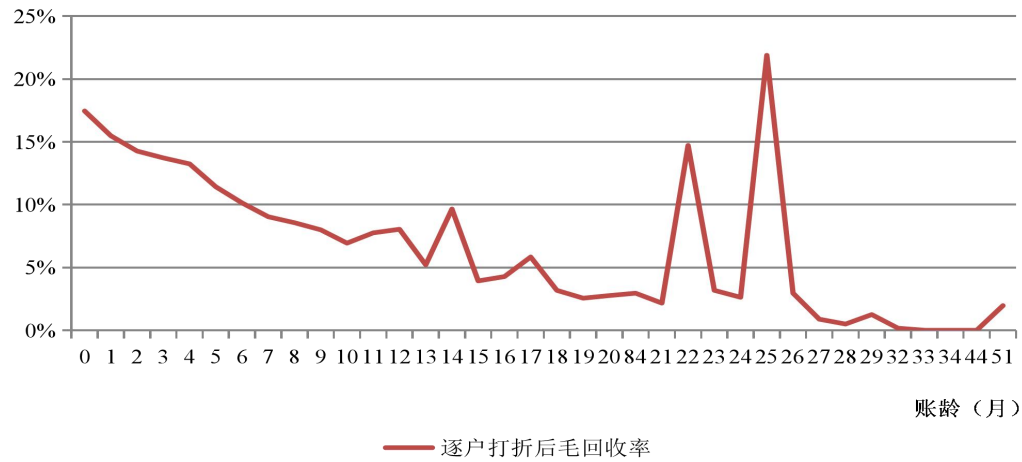
信用卡透支资产池的账龄与回收率的关系图
